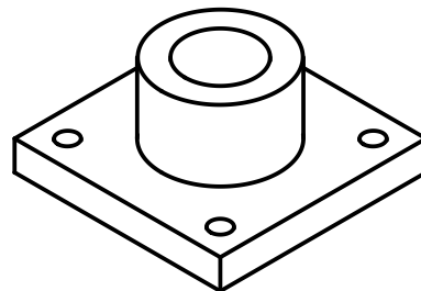
VISTA ISOMÉTRICA 1:2
